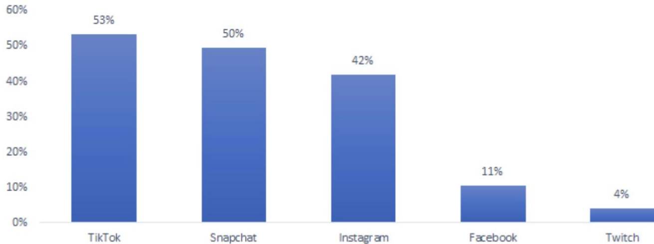
Daglig räckvidd bland 9-19-åringar
